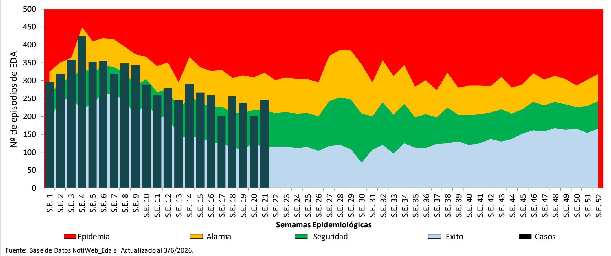
CANAL ENDÉMICO DE EPISODIOS DE EDA SEGÚN SEMANAS EPIDEMIOLÓGICAS ( SIN AÑOS DE PANDEMIA 2020 - 2022 ) RED INTEGRADA DE SALUD HUAURA OYÓN, 2026 A LA S.E. 21
