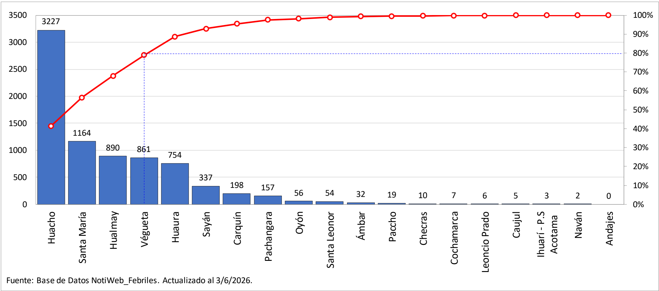
DIAGRAMA DE PARETO PARA EL ANÁLISIS DE FEBRILES SEGÚN DISTRITOS. RED INTEGRADA DE SALUD HUAURA OYÓN, 2026 A LA S.E. 21
