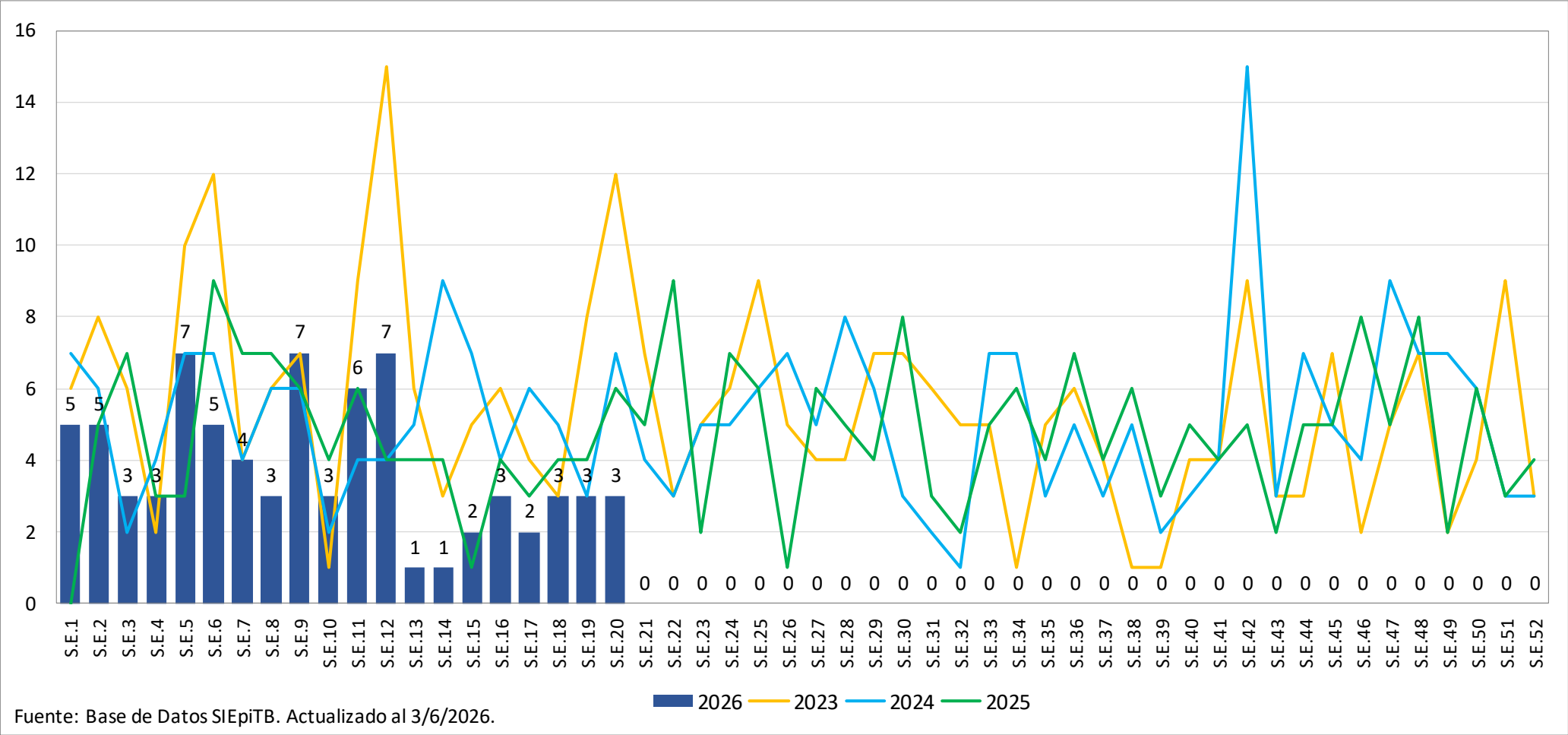
TENDENCIA DE CASOS NOTIFICADOS DE TUBERCULOSIS SEGÚN SEMANA EPIDEMIOLÓGICA RED INTEGRADA DE SALUD HUAURA OYÓN, 2023 - 2026 A LA S.E. 21
