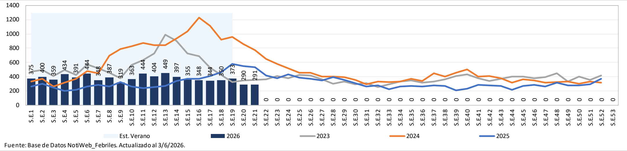
TENDENCIA Y ANÁLISIS DE FEBRILES SEGÚN AÑOS Y SEMANA EPIDEMIOLÓGICA RED INTEGRADA DE SALUD HUAURA OYÓN, 2023 - 2026 A LA S.E. 21
