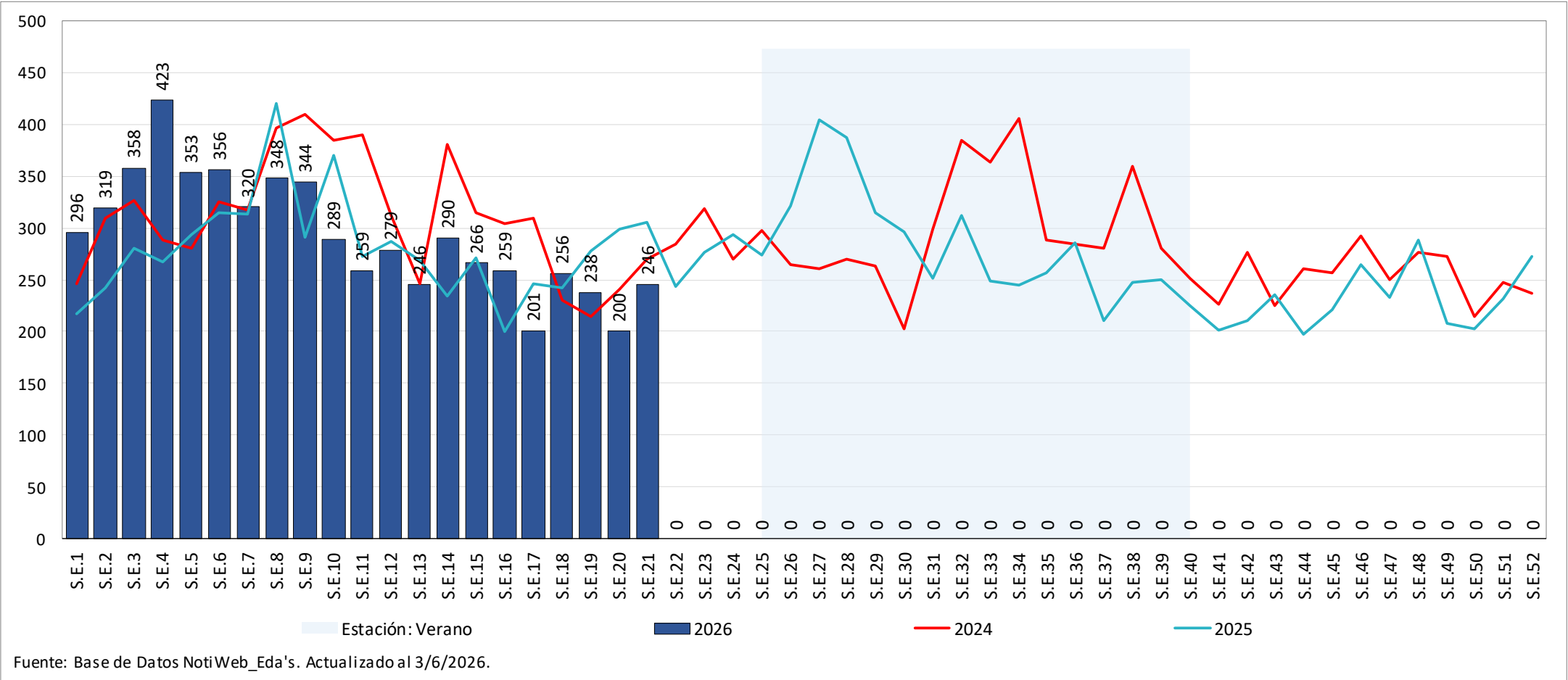
TENDENCIA DE NÚMERO DE EPISODIOS DE EDA SEGÚN SEMANAS EPIDEMIOLÓGICAS RED INTEGRADA DE SALUD HUAURA OYÓN, 2024 - 2026 A LA S.E. 21
