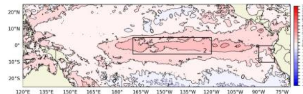
Figura 1. Promedio (del 27 de diciembre de 2023 al 09 de enero de 2024) de las anomalías de la TSM en el Pacífico tropical. Las regiones Niño 3.4, en el centro del Pacífico, y Niño 1+2, frente a la costa peruana, están delimitadas con recuadros de color negro. Fuente: OSTIA.
